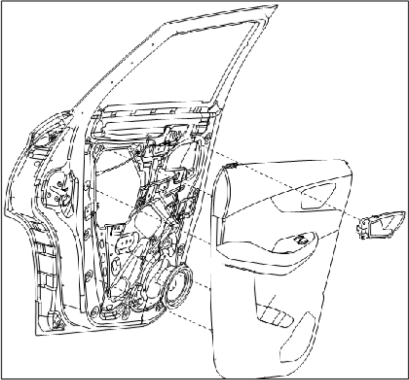
电动车窗部件视图（后门）
